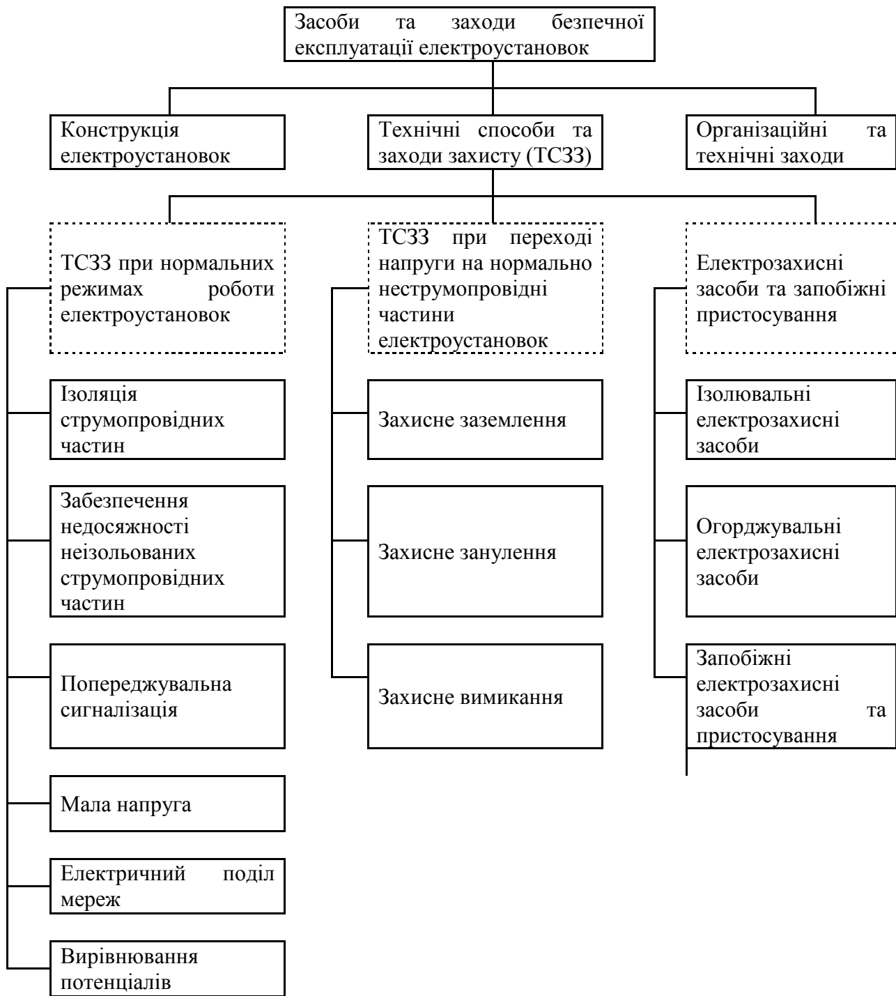
Рис. 8. Класифікація засобів та заходів безпечної експлуатації електроустановок
