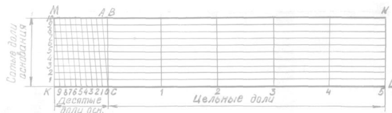
Рис. 5. Масштаб поперечний
