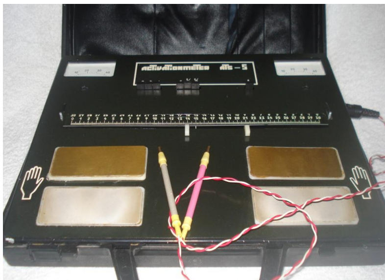
Рис. 40. Пристрій «Активометр АЦ-5»
