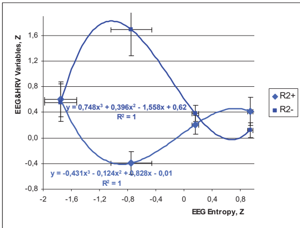
Рис. 7.2. Друга пара патернів параметрів EEG та ВСР за різних рівнів ентропії EEG
