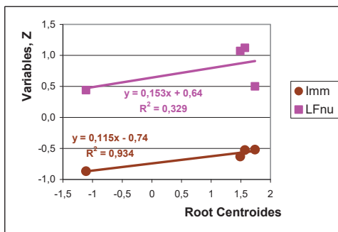
Рис. 8.8. Нормалізовані значення LFnu та імуних параметрів, ущільнених в третьому корені, які корелюють з ним позитивно
