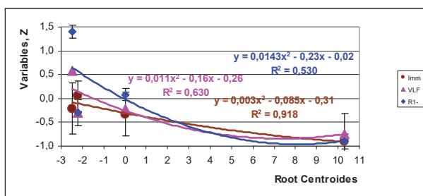
Рис. 8.4. Нормалізовані значення ( Z \pm SE ) ЩСП θ-ритму , VLF та імуних параметрів, конденсованих у першому корені, які негативно корелюють з ним
