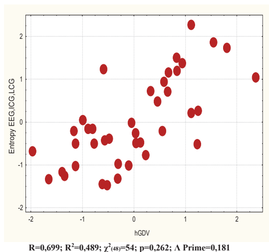
Рис. 11.4. Точковий графік канонічної кореляції між ентропією ГРВ-грами (вісь X) та ЕЕГ, ЛЦГ і ЦЦГ (вісь Y)
