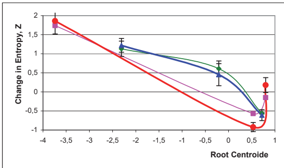
Рис. 9.7. Патерни інтегральних змін ентропії для першого і другого коренів
