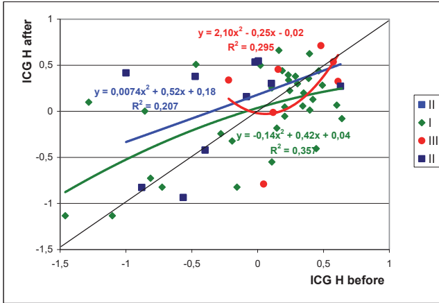
Рис. 9.15. Нормалізовані середні рівні ентропії імуноцитограми до (вісь X) і після (вісь Y) бальнеотерапії у членів різних кластерів
