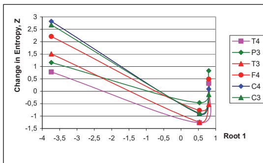
Рис. 9.5. Патерни змін ентропії ЩСП в локусах EEG, які репрезентують перший корінь
