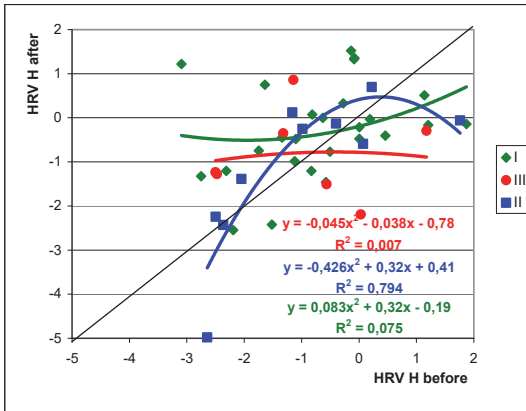
Рис. 9.13. Нормалізовані середні рівні ентропії ВРС до (вісь Х) і після (вісь Y) бальнеотерапії у членів різних кластерів
