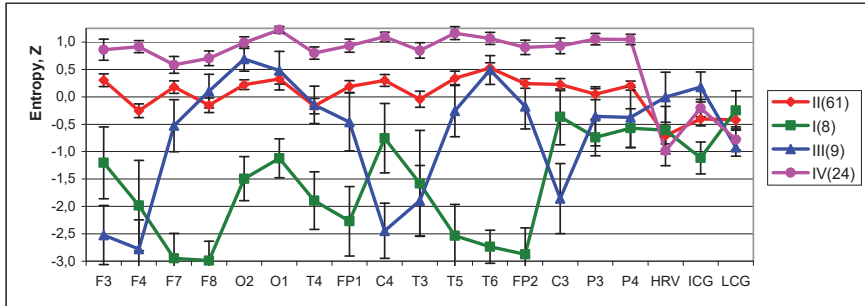
Рис. 6.2. Z-оцінки ( M \pm SE ) ентропії ЩСП в локусах EEG, ВРС, ЛЦГ та ЦГ у членів різних кластерів
