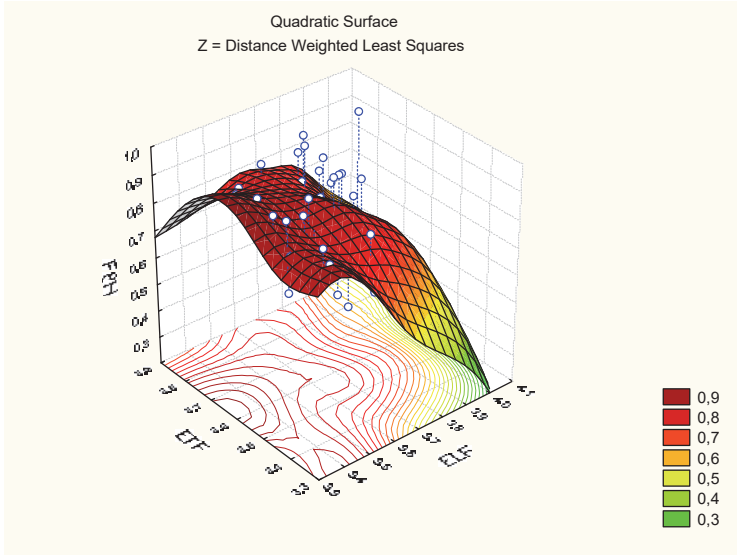
Рис. 11.2. Точковий графік залежності ентропії ЩСП ЕЕГ в локусі F8 (вісь Z) від ентропій ГРВ-грами (відфільтрованої) в лівій (вісь X) та фронтальній (вісь Y) проекціях
