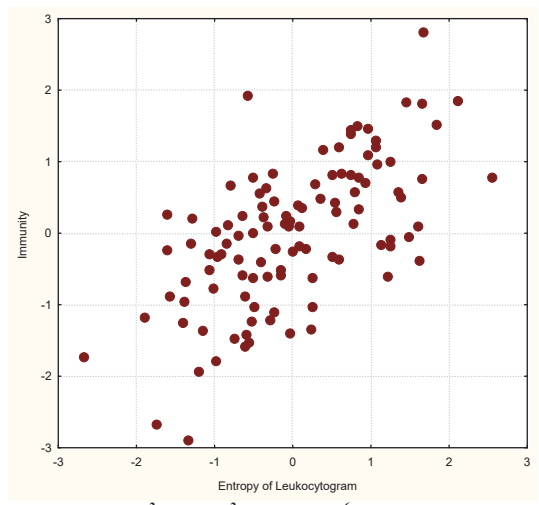
Рис. 3.18. Точковий графік канонічної кореляції між ентропією лейкоцитограми (лінія X) та параметрами імунітету (лінія Y)
