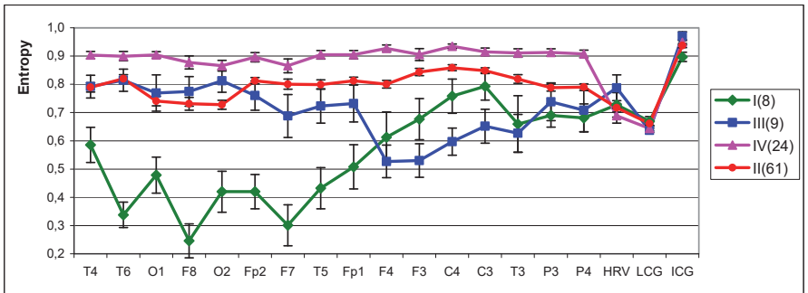
Рис. 6.1. Фактичні середні значення ( M \pm SE ) ентропії ЩСП в локусах ЕЕГ, а також ВРС, ЛЦГ та ЦГ у членів різних кластерів
