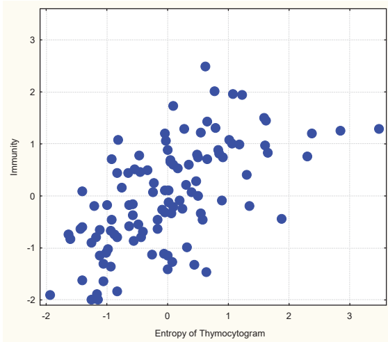
Рис. 3.15. Точковий графік канонічної кореляції між ентропією тимоцитограми (лінія X) та параметрами імунітету (лінія Y)
