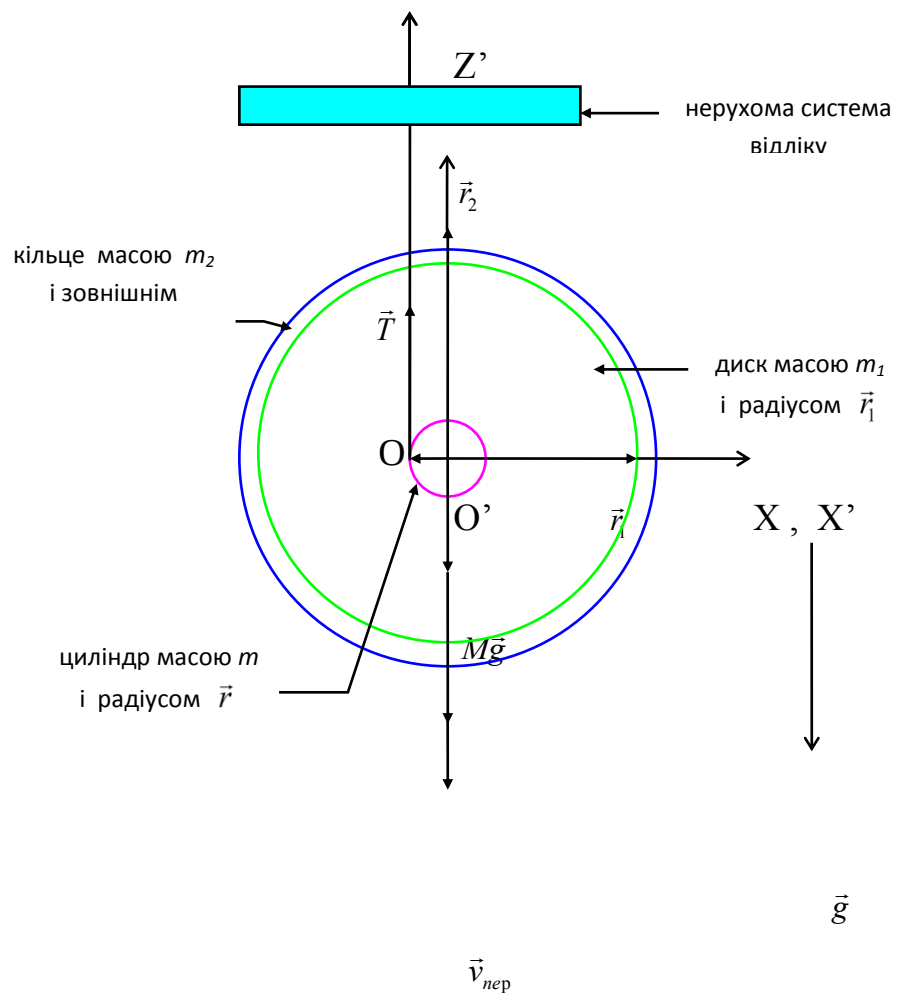
Рис. 9. Маятник Максвела (на початку опускання)
