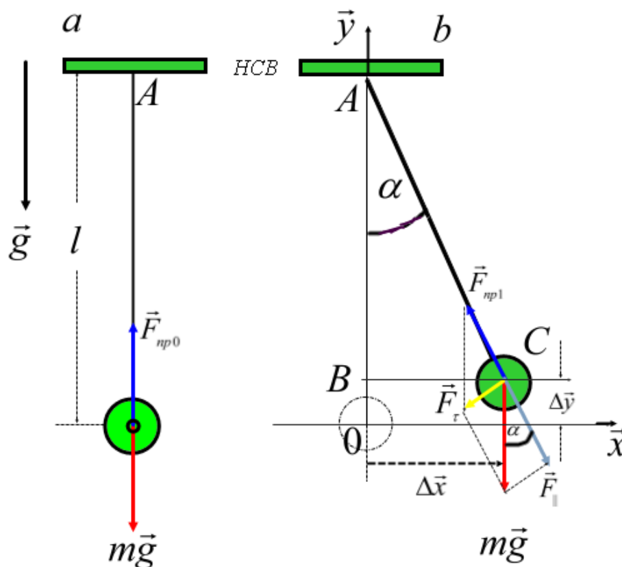
Рис.5. Математичний маятник
