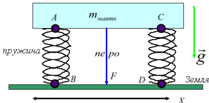
Рис.14. Схема сейсмографа
