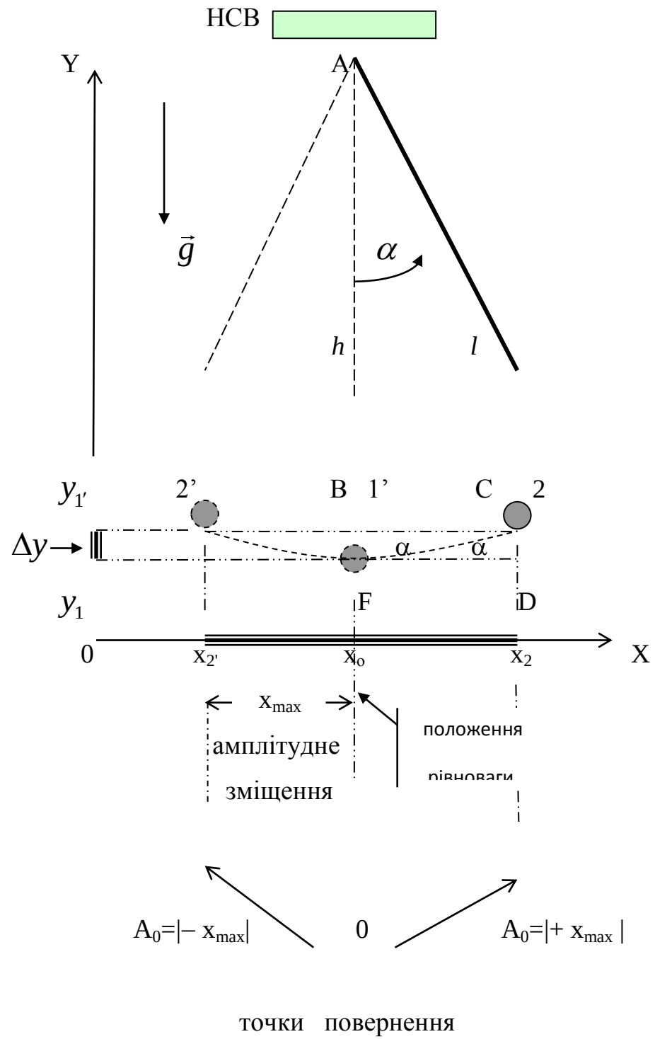
Рис.5с. Математичний маятник
