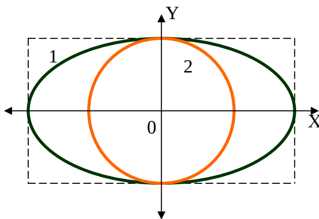
Рис. 5. Еліпс (коло), симетричний відносно системи координат
