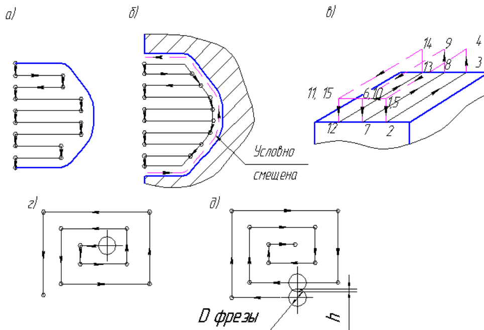
Рис. 7. Типові схеми фрезерних проходів: а - зигзагоподібна без обходу контуру; б - зигзагоподібна з проходом уздовж кордонів наприкінці обробки; в - зигзагоподібна Ш-образного типу; г – спиралевидний рух інструмента від центру області до периферії; д - спиралевидний рух інструмента від периферії до центру області.
