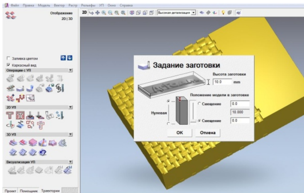
Рис. 4.16. Завдання параметрів заготовки для обробки на верстті
