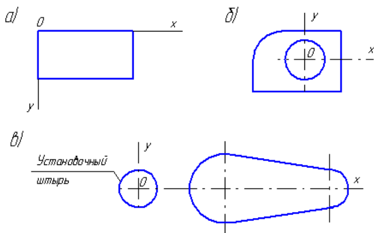
Рис. 1. Приклади вибору початку координат деталі:
